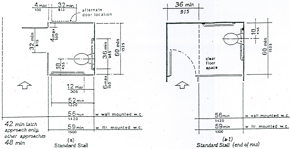
Fig. 30 Toilet Stalls
